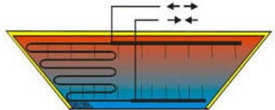
Bild: Bauart eines erdvergrabenen Kies-Wasser-Behälters ohne tragende Außenwand, als Beispiel für ein neues Behälterkonzept für Eisspeicher (Quelle: ISBN 3-9805274-2-5)
